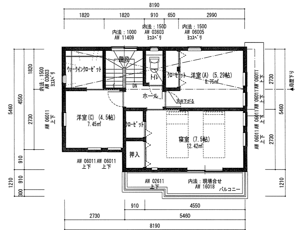
2階平面図 (プレゼン) 1/100
