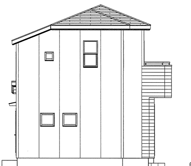
西立面図 1/100
