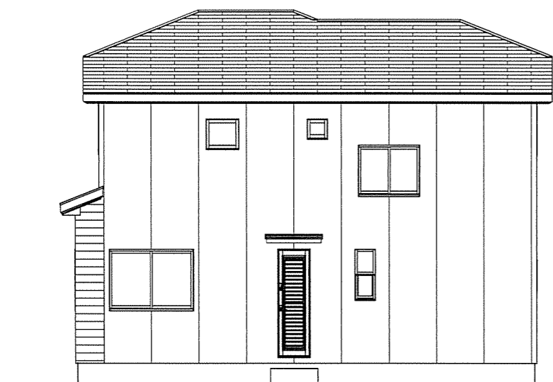
北立面図 1/100
